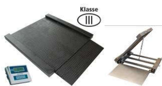
KPZ 2D
