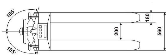
Rozměry v mm
