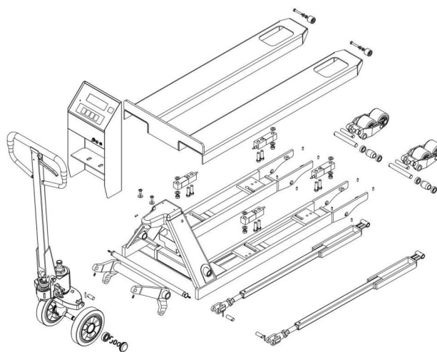
KPZ 71-9 / Paletový vozík s váhou
