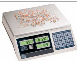
KPZ 2-04(E)-3 M Počítačí váha robustní průmyslové provedení
